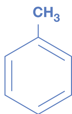
Metil-benzene (toluene)
