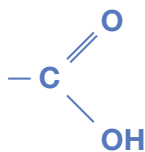
Gruppo carbossile
