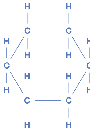
Cicloesano
