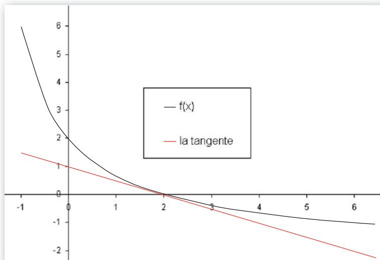
▲ Figura 2 Il grafico della f(x) e della tangente in T(2; 0) .
