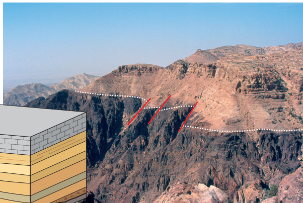
DISCORDANZA SEMPLICE
