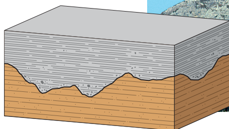
DISCONFORMITÀ
