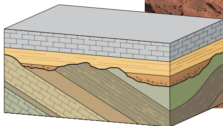
DISCORDANZA ANGOLARE
