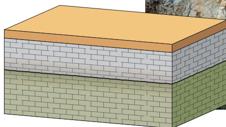
PARACONCORDANZA
