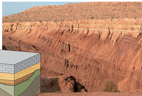
DISCORDANZA ANGOLARE
