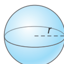
sfera
