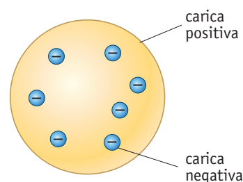
▲ Figura 1 Rappresentazione del modello atomico di Thomson.
