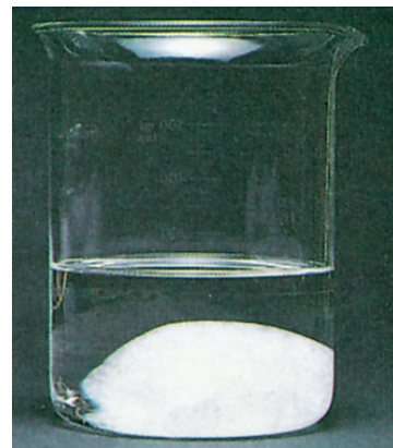
► Figura A Durante la solidificazione i cristalli di benzene, avendo densità maggiore, affondano nel liquido.
