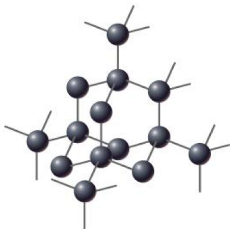
diamante
