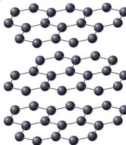
grafite
