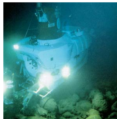
▲ 2 Ecco come è apparso il fondo dell'Atlantico all'equipaggio di uno dei piccoli sottomarini appositamente progettati per ricerche oceanografiche. L'immersione cui si riferisce questa foto è stata effettuata in corrispondenza della Dorsale Medio-atlantica, lungo la quale da numerose fessure fuoriescono grandi quantità di lave, che, a contatto con le fredde acque dell'oceano, si solidificano, assumendo una caratteristica struttura in masse tondeggianti. Le rocce che in tal modo si formano sono basalti, e rocce analoghe costituiscono il «pavimento» di tutti gli oceani. Così è nata, oltre 100 milioni di anni fa, anche la roccia della nostra storia. (Woods Hole Oceanographic Inst. Ma., USA)
