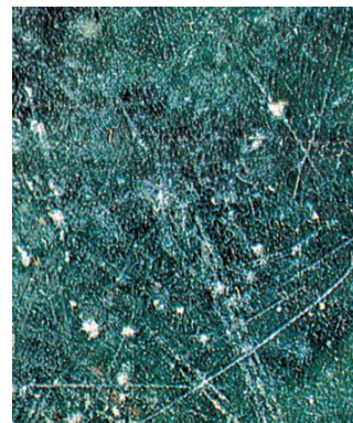
▲ 1 Sottili strie sulla superficie di un ciottolo di origine «glaciale» (a destra, un dettaglio). Esso ha subito un trasporto ad opera di un ghiacciaio, prima di entrare a far parte del materiale di una morena. (L. Spinozzi)
