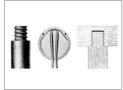
Disegno del collegamento mediante filettatura tra zampe e telaio del sedile nelle sedie Thonet (da catalogo originale).
