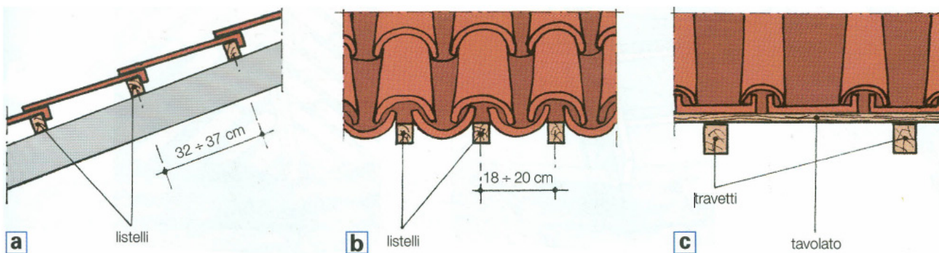
Interasse dei listelli per la posa di tegole a innesto (a), coppi (b) e su tavolato per copertura alla romana (c).
