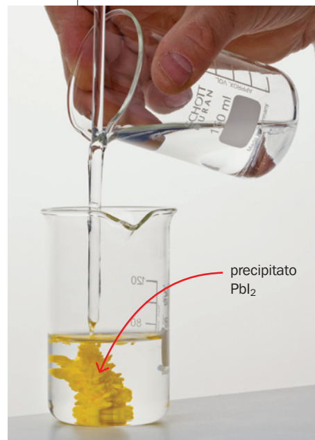
▲ Figura 1 Le soluzioni dei due sali sono entrambe incolori e contengono gli ioni resi liberi in seguito al processo di dissociazione ionica. Versando una soluzione nell'altra si forma una sostanza insolubile di colore giallo.
