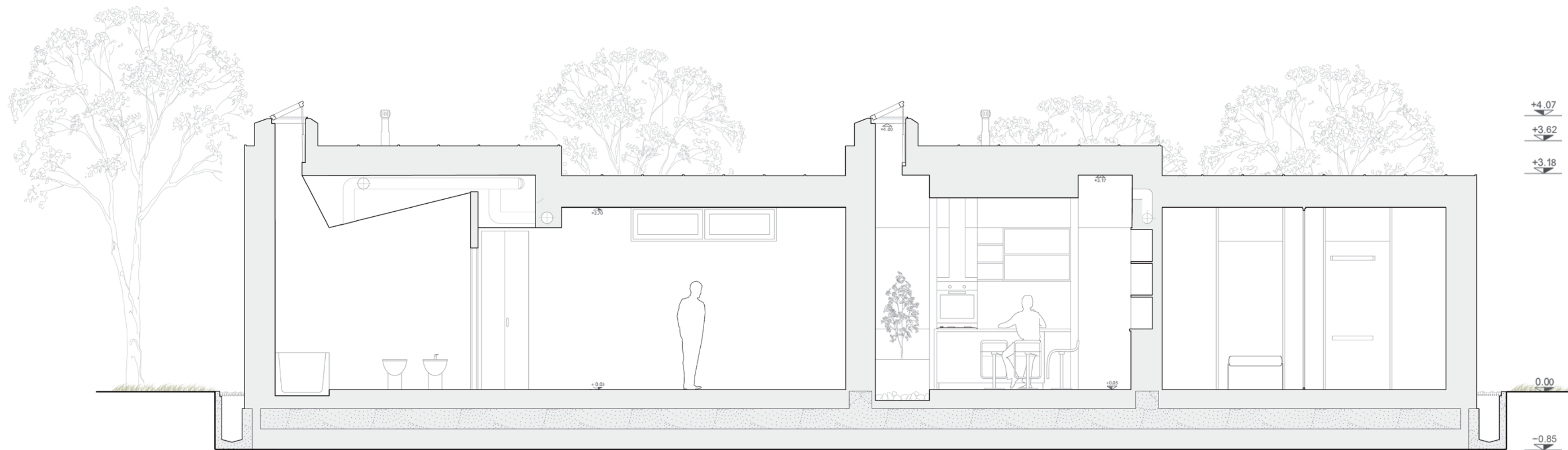
sezione a-a scala 1:50
