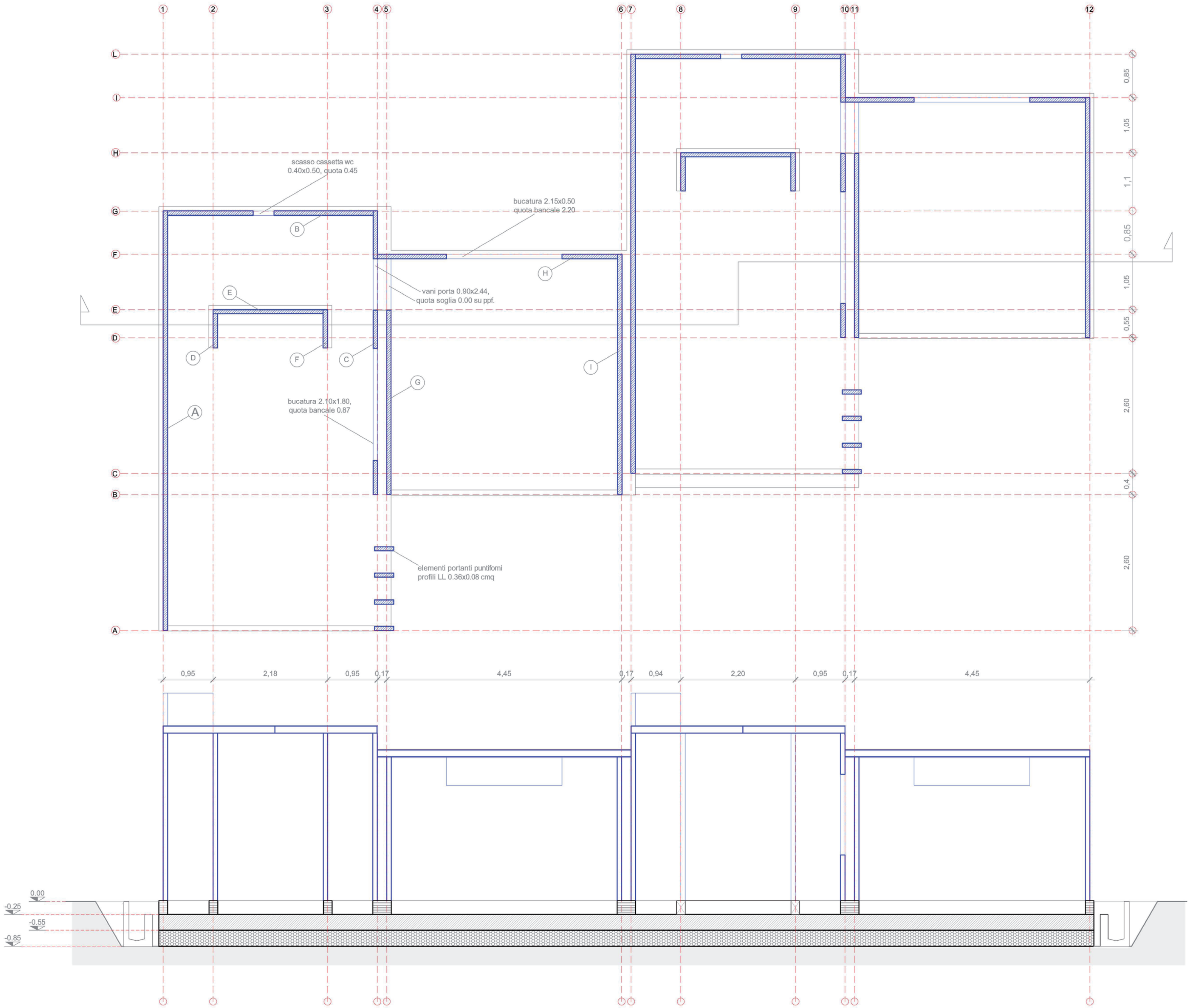
struttura in elevazione orizz. e vert. a pannelli Rasom - scala 1:50
