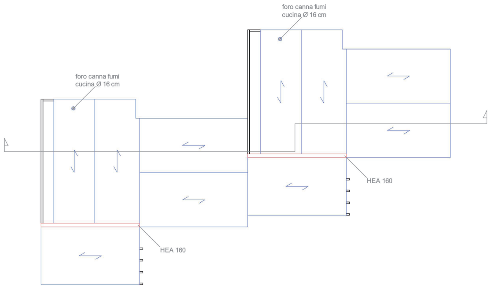
struttura orizzontale di copertura in pannelli LenoTec - scala 1:100
