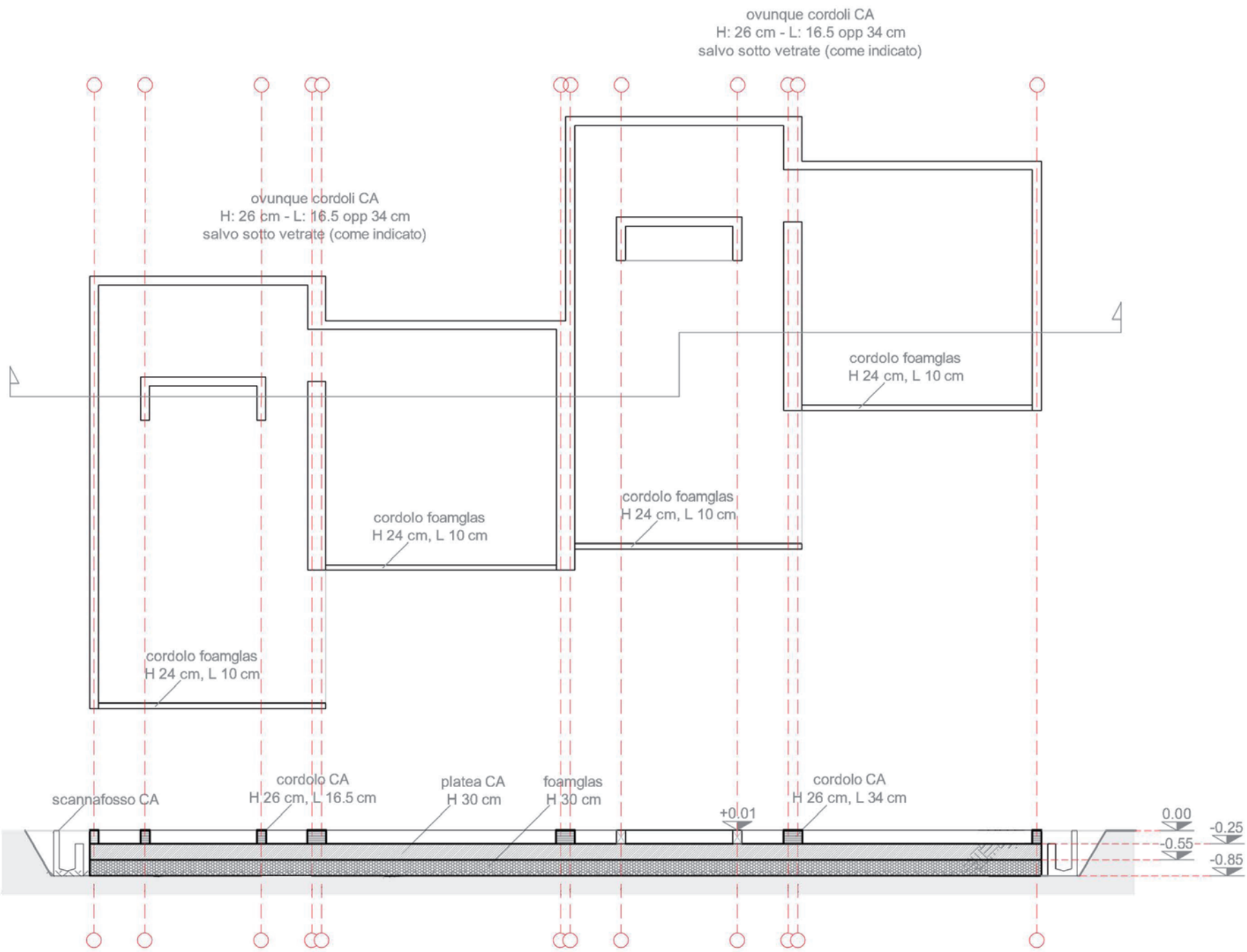
opere fondali in CA * - scala 1:100 * trattasi di CLS debolmente armato, saltuariamente sostituito da vetro cellulare
